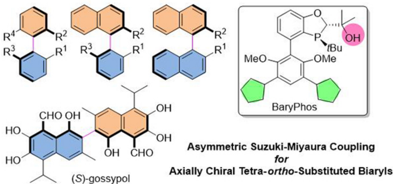
图1 不对称偶联促进轴手性邻位四取代联芳基化合物的高效合成
