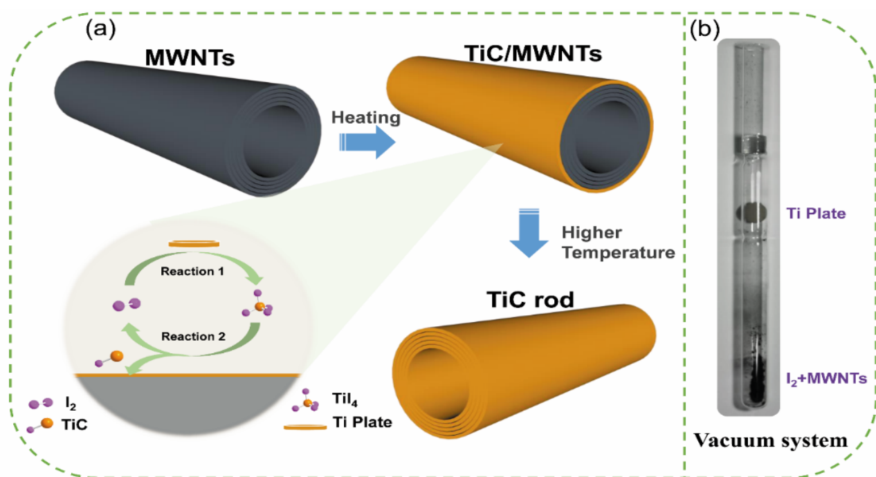
碳/非碳复合正极载体材料制备过程
