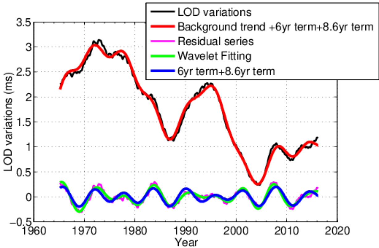
图1. 利用本文所提方法(NMWT+BEPME)提取的日长亚十年振荡结果（红线）与原始信号（黑线）的比较：两曲线总体上非常吻合，表明日长亚十年变化特征可以很好的由6年和8.6年两种频率信号的叠加解释
