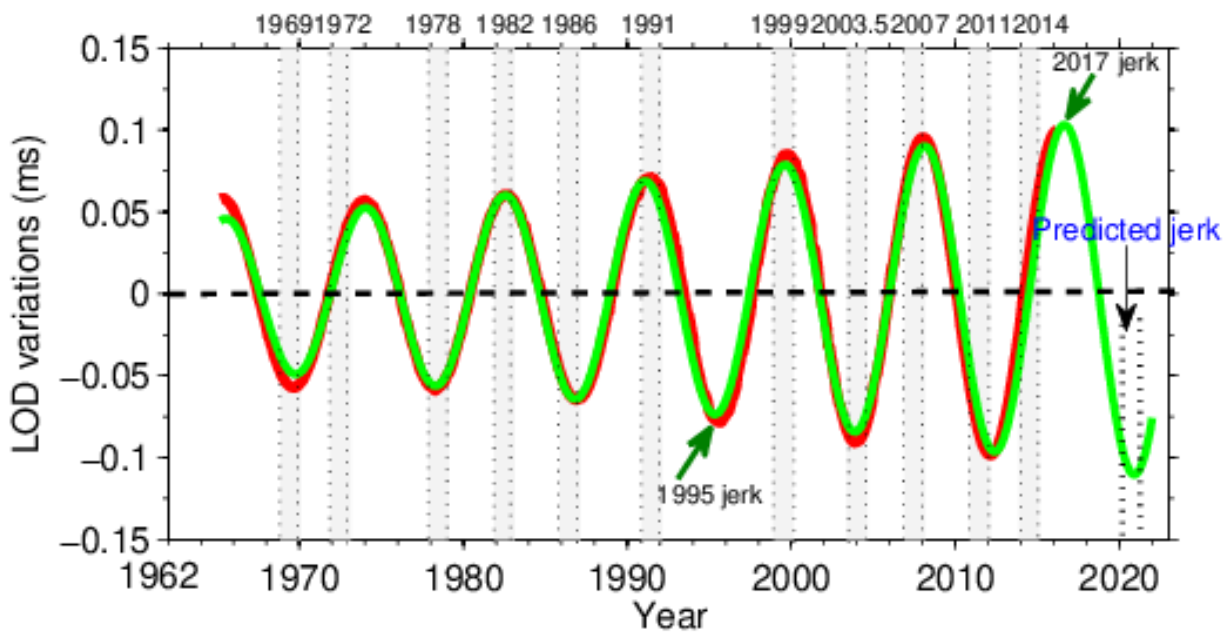
图2. 本文恢复的目标8.6年周期振荡与地磁急变(jerks)时刻(阴影矩形条带)所示的对应关系；红色曲线是本文恢复的结果，绿线是红线的最小二乘拟合结果，该结果可进一步用于预测未来jerk发生
