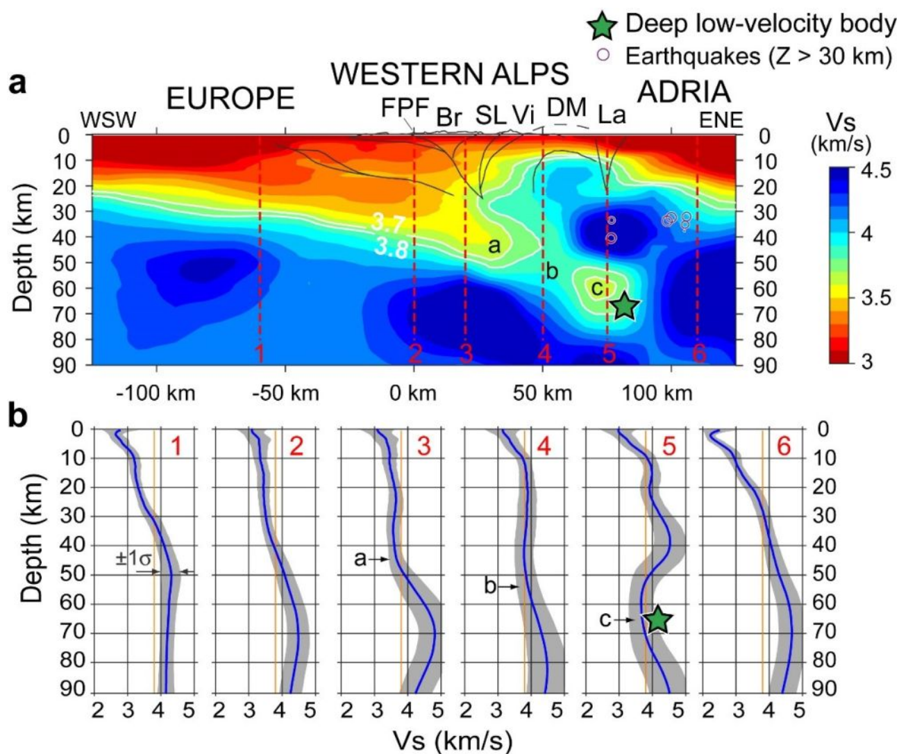
图2 沿着中-意-法西阿尔卑斯地震观测线的横波速度分布。(a)速度横截面；(b)典型控制点下方的速度剖面。绿色五角星显示低速层的位置
