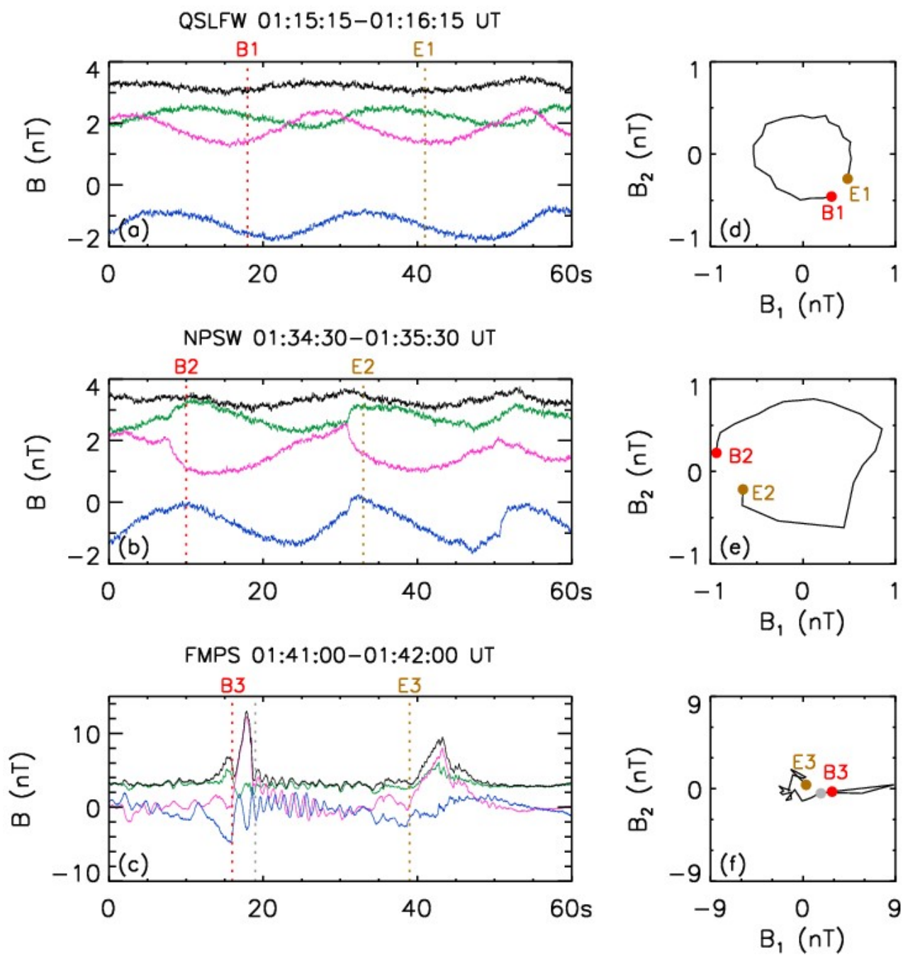
图2 激波形成过程中三个典型瞬间
