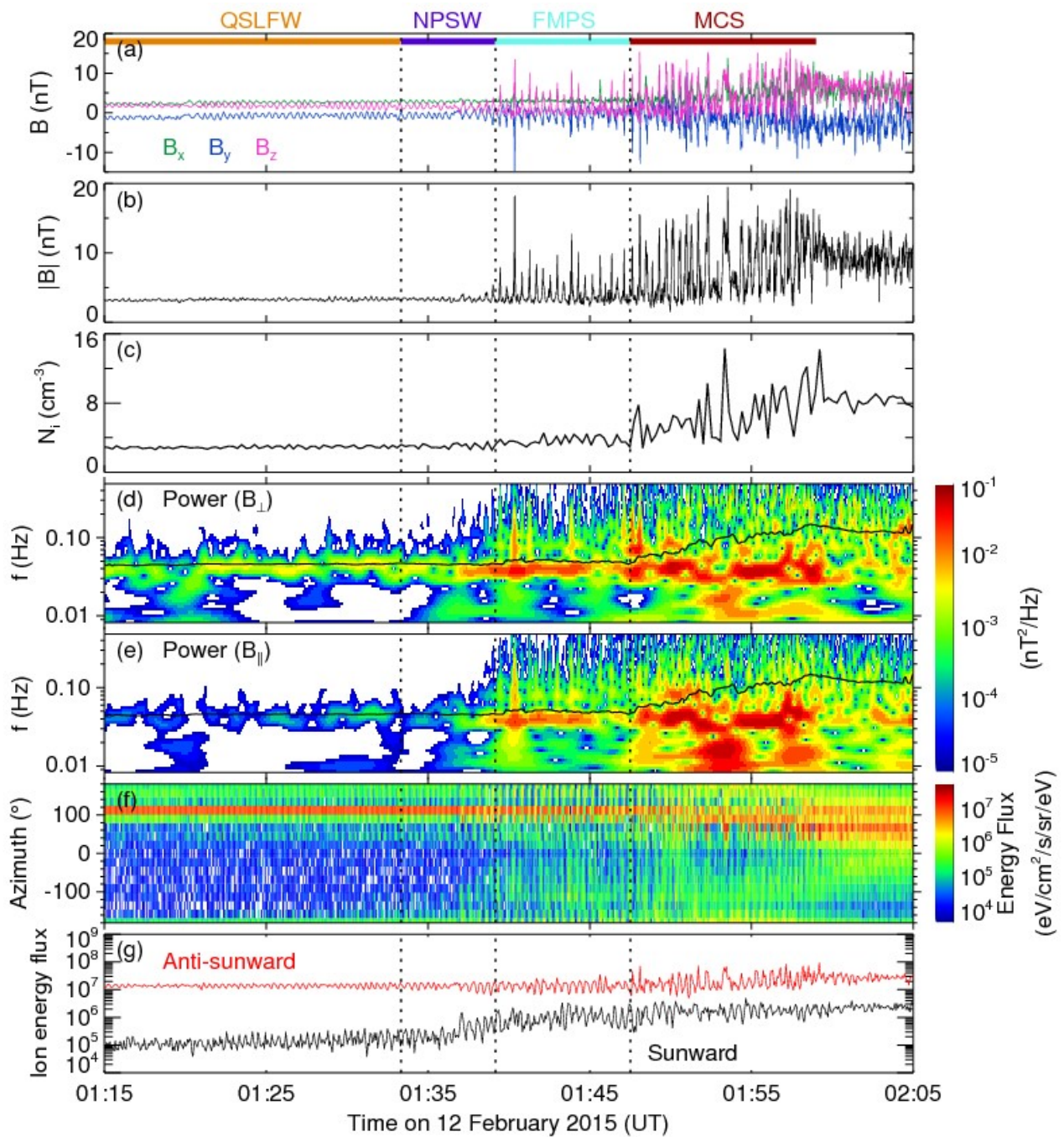
图1 波动演化成周期性激波的完整序列。(a, b) 磁场三分量和总场；(c) 离子数密度；(d, e) 磁场功率谱；(f) 仪器坐标系下离子方位角分布；(g) 离子能通量
