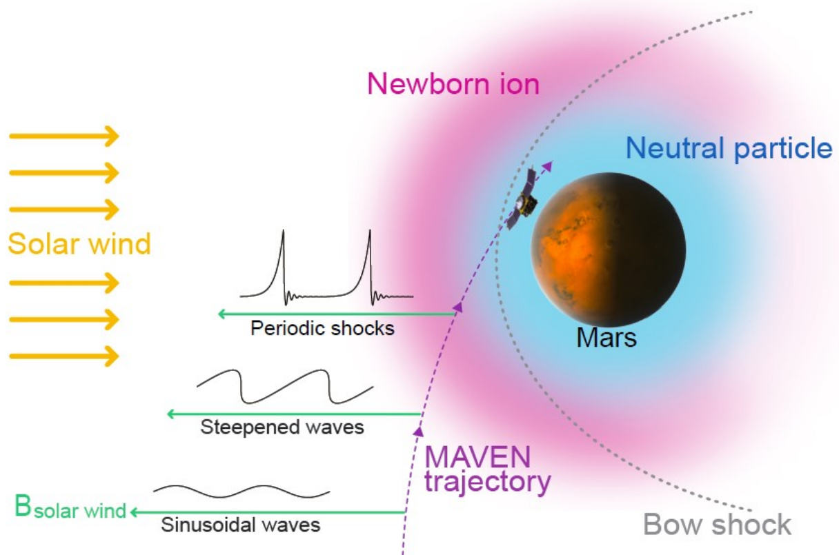
图3 火星空间环境中周期性激波由波动演化的示意图
