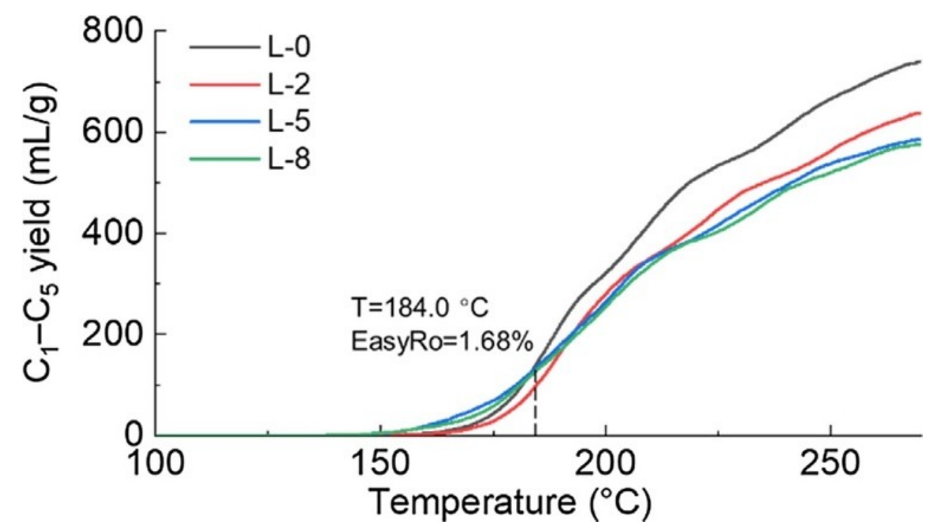
图1. 通过生烃动力学模拟得到的不同程度生物降解原油L-x在地质条件下（2 /Ma）的烃类气体产率(x=0, 2, 5, and 8，x为生物降解的PM等级，L-0级为未降解，L-2级为轻度降解，L-5级为重度降解，L-8级为严重降解)。
