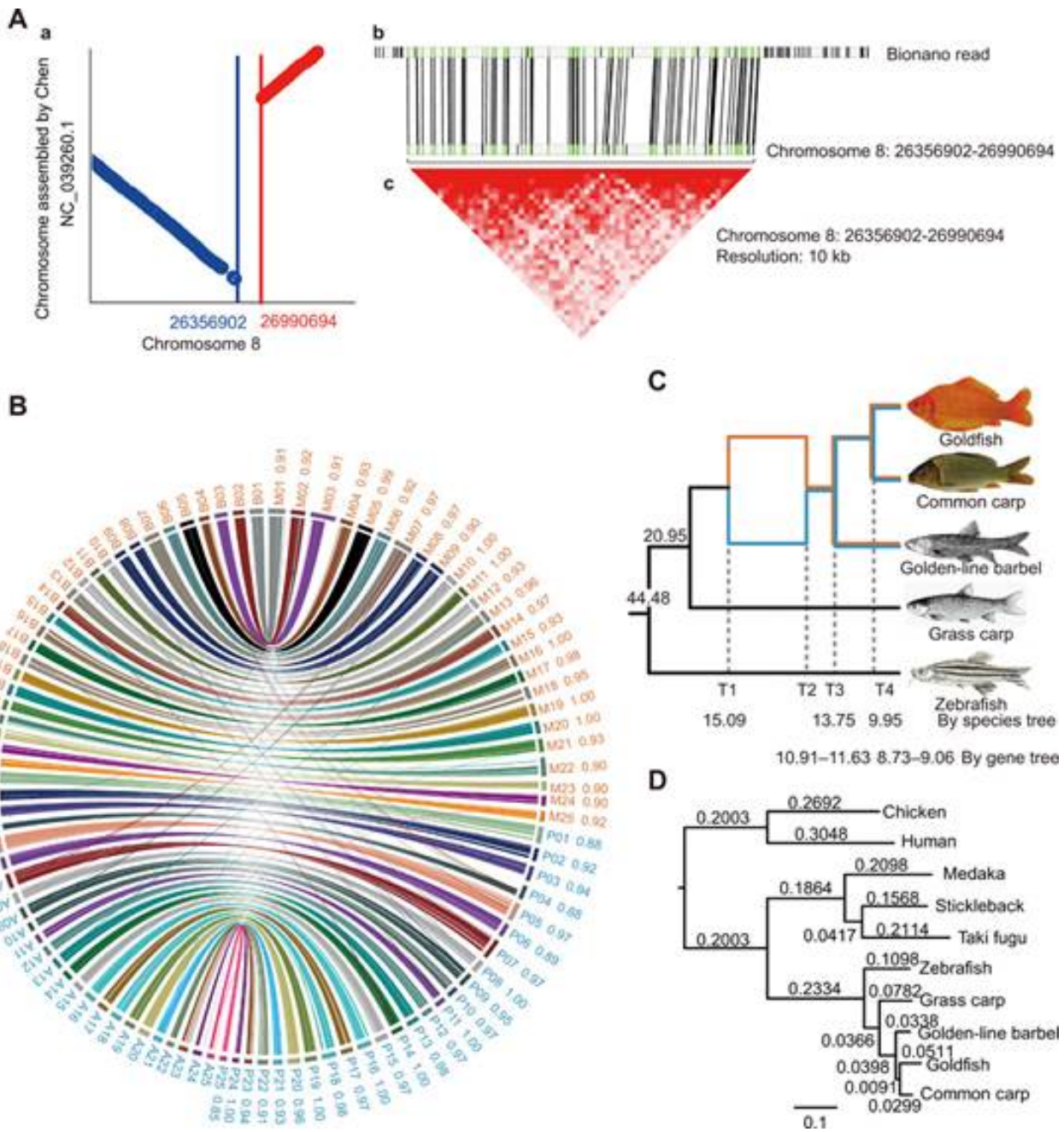
图：红鲫基因组组装质量比较、共线性及鲤亚科鱼类多倍化演化历史重建。(A)红鲫基因组组装质量；(B)红鲫与鲤鱼的亚基因组共线性分析结果；(C)基于系统发育关系重建鲤亚科基因组的异源多倍化演化历史；(D)基于单拷贝直系同源基因构建的物种树。
