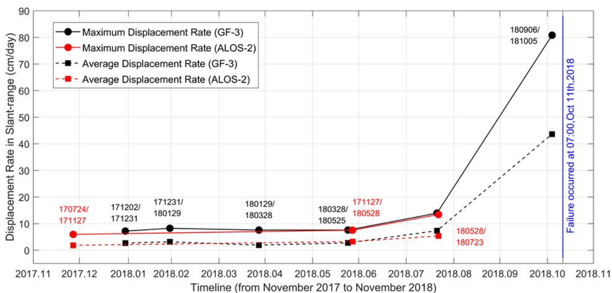
金沙江滑坡时间位移模式
