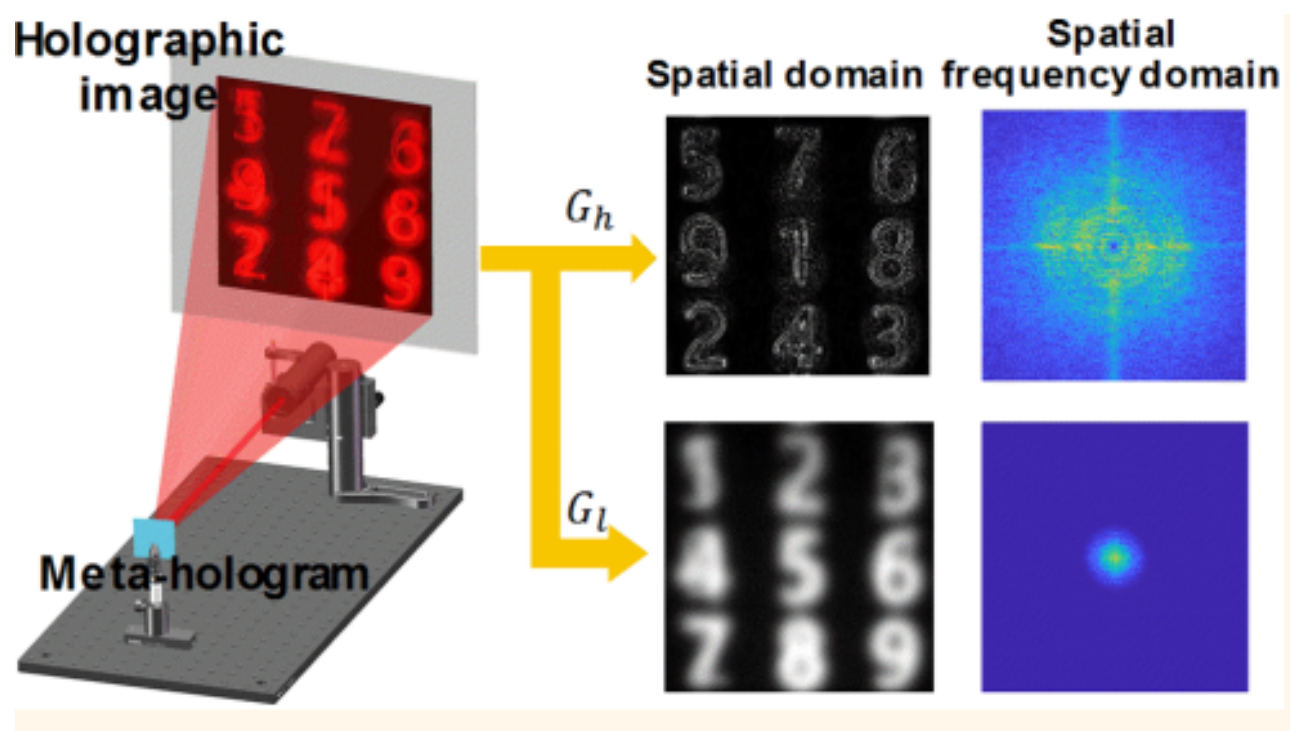
图1 超表面空间频率复用技术示意图和测试结果
