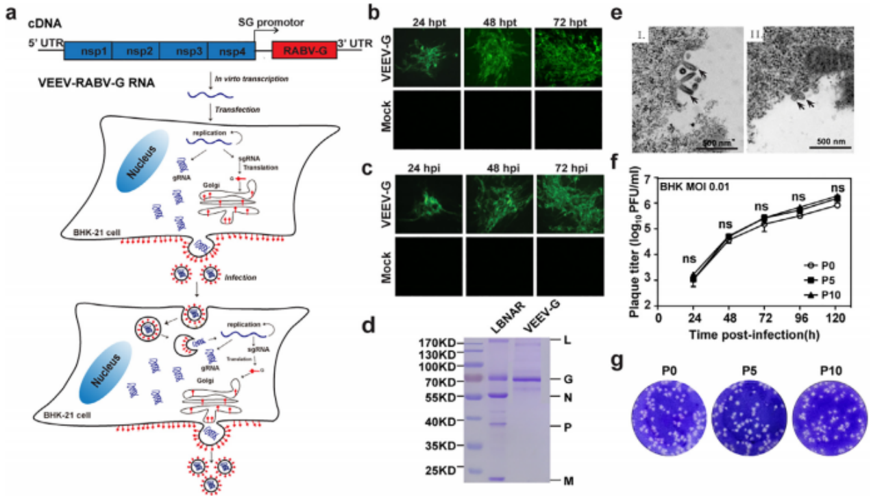
图1. VEEV-RABV-G重组病毒鉴定。a：VEEV-RABV-G重组病毒产生及感染示意图；b：VEEV-RABV-G转染细胞后不同时间点IFA检测；c：VEEV-RABV-G病毒感染细胞后不同时间点IFA检测；d：纯化的VEEV-RABV-G重组病毒和LBNAR病毒SDS-PAGE电泳分析；e：VEEV-RABV-G和LBNAR感染细胞后电镜观察；f：传代后的病毒生长曲线比较；g：传代后的病毒噬斑比较。
